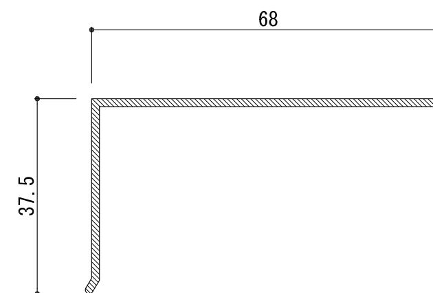
0-18B 内ジョイント W=50
